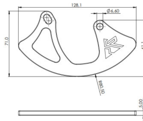
36 zubů
