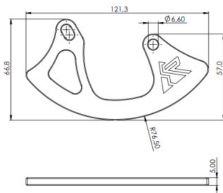
34 zubů
